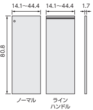
品名: ARNC扉オーダー9015~90 サイズ: W14.1~44.4×D1.7×H80.8cm (1枚あたり) 特長: 高さ: 本体88.1cmに対応
