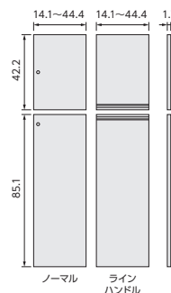
品名: ARNC扉オーダー1415~90 サイズ: W14.1~44.4×D1.7× 上: H42.2cm/下: H85.1cm (1枚あたり) 特長: 高さ: 本体135cmに対応
