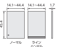
品名: ARNC突っ張り棚用扉オーダー 4115~90 サイズ: W14.1~44.4×D1.7×H45.4cm (1枚あたり) 特長: 高さ突っ張り高さ41cmに対応
