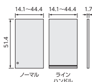
品名: ARNC突っ張り棚用扉オーダー 4715~90 サイズ: W14.1~44.4×D1.7×H51.4cm (1枚あたり) 特長: 高さ突っ張り高さ47cmに対応
