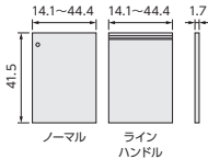
品名: ARNC扉オーダー5015~90 サイズ: W14.1~44.4×D1.7×H41.5cm (1枚あたり) 特長: 高さ本体49cmに対応
