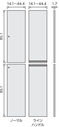
品名: ARNC扉オーダー1815~90 サイズ: W14.1~44.4×D1.7× 上: H85.1cm/下: H85.1cm (1枚あたり) 特長: 高さ本体178cmに対応
