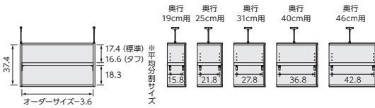
品名: ARNC突っ張り棚41オーダー ※イラストタイプ
