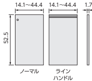
品名: ARNC扉オーダー6015~90 サイズ: W14.1~44.4×D1.7×H52.5cm (1枚あたり) 特長: 高さ本体60cmに対応
