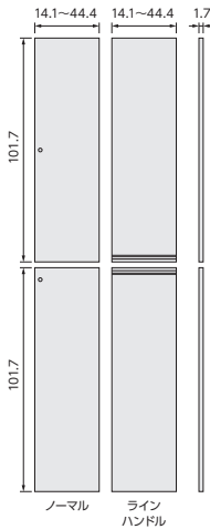
品名: ARNC扉オーダー2115~90 サイズ: W14.1~44.4×D1.7× 上: H101.7cm/下: H101.7cm (1枚あたり) 特長: 高さ本体211.1cmに対応
