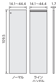
品名: ARNC扉オーダー1215~90 サイズ: W14.1~44.4×D1.7×H109.5cm (1枚あたり) 特長: 高さ: 本体117cmに対応
