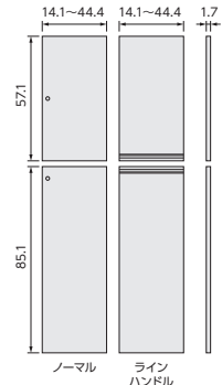
品名: ARNC扉オーダー1515~90 サイズ: W14.1~44.4×D1.7× 上: H57.1cm/下: H85.1cm (1枚あたり) 特長: 高さ: 本体149.9cmに対応
