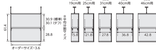
品名: ARNC突っ張り棚65オーダー ※イラストタイプ
