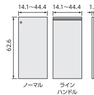
品名: ARNC扉オーダー7015~90 サイズ: W14.1~44.4×D1.7×H62.6cm (1枚あたり) 特長: 高さ本体70cmに対応
