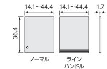
品名: ARNC突っ張り棚用扉オーダー 3215~90 サイズ: W14.1~44.4×D1.7×H36.4cm (1枚あたり) 特長: 高さ突っ張り高さ32cmに対応
